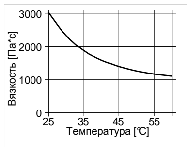
Диаграмма 1 Вязкость SikaPower®-4591
